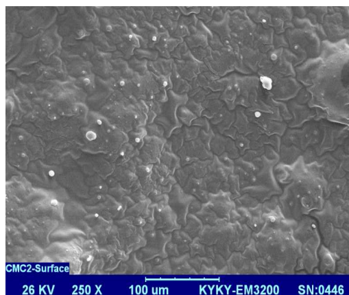
شکل ۹ تصویر سطح نان پوشش داده شده با کربوکسی متیل سلولز پس از ۳ روز نگهداری
