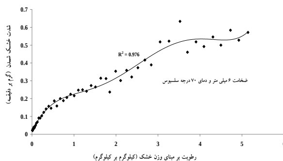
شکل ۹ آهنگ خشک شدن ورقه‌های نازک سیب‌زمینی با ضخامت ۶ میلی‌متر، الف- دما ۵۰ °C، ب- دما ۶۰ °C، ج- دما ۷۰ °C
