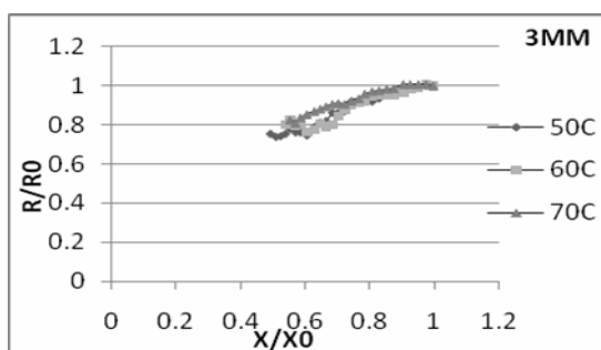
شکل ۱۳ تغییرات کرویت (قطر بزرگ در جهت باد)
