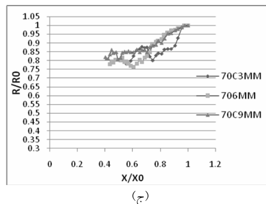
شکل ۱۵ تغییر کرویت با کاهش رطوبت، ج- دما ۷۰ °C
