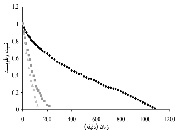
شکل ۹ روند خشک شدن نمونه‌های تیمار شده ( P_2 )
