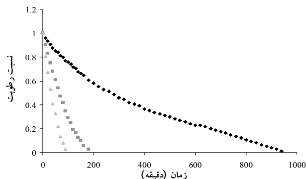
شکل ۱۰ روند خشک شدن نمونه‌های تیمار شده ( P_2 )
