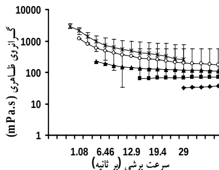
شکل ۳ نمایش تأثیر سرعت برشی روی گرانروی محلولهای صمغ کتیرای ایرانی در غلظتهای مختلف (۱، ۲، ۳، ۴، ۵)؛ *، O، ▲، ■، ◆؛ ۱، ۲، ۳، ۴، ۵، پ هاش ثابت ۷ و دمای ۲۵ درجه سانتی‌گراد.
