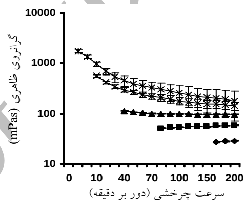
شکل ۲ نمایش ارتباط سرعت چرخشی و گرانروی محلولهای صمغ کتیرای ایرانی در غلظتهای مختلف (♦، ۱؛ ■، ۲؛ ▲، ۳؛ ○، ۴؛ *، ۵) (الف) دما ۲۵ درجه سانتی گراد، پ هاش ۴ ب) دما ۲۵ درجه سانتی گراد، پ هاش ۷ ج) دما ۲۵ درجه سانتی گراد، پ هاش ۱۰ د) دما ۵۵ درجه سانتی گراد، د هاش ۴ ه) دما ۵۵ درجه سانتی گراد، پ هاش ۷ و) دما ۵۵ درجه سانتی گراد و پ هاش ۱۰.
