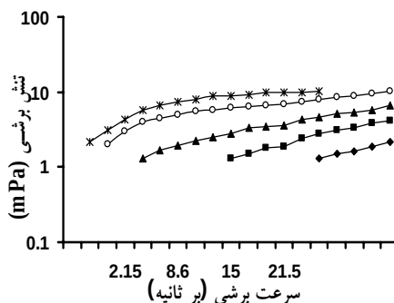
شکل ۴ رفتار جریان محلولهای صمغ کتیرای ایرانی در غلظتهای مختلف (۱، ۲، ۳، ۴، ۵)؛ *، O، ▲، ■، ◆؛ ۱، ۲، ۳، ۴، ۵، پ هاش ثابت ۷ و دمای ۲۵ درجه سانتی‌گراد.
