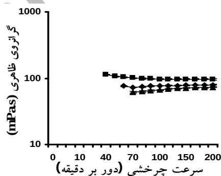
شکل ۵ نمایش ارتباط سرعت چرخشی و گرانروی محلول ۳ گرم در لیتر صمغ کتیرای ایرانی در پهاش‌های مختلف (۴، ۷، ۱۰). (الف) دما ۵ درجه سانتی‌گراد (ب) دما ۲۵ درجه سانتی‌گراد (ج) دما ۵۵ درجه سانتی‌گراد.
