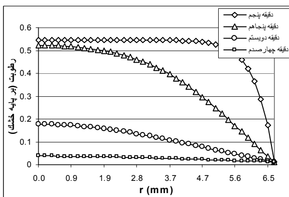
کل ۷- تغییرات رطوبت از مرکز به سطح دانه با رطوبت اولیه ۵۴/۶۲٪، دمای 70^{\circ}\text{C} و ضریب پخش رطوبت ( 7/5 \times 10^{-11} \text{ m}^2/\text{s} )
