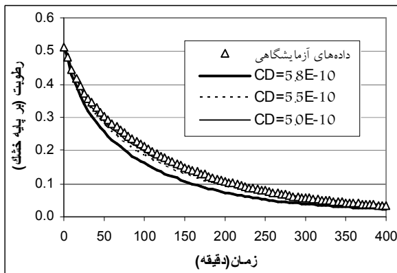
شکل ۳ - تغییر رطوبت در طی خشک شدن پسته با رطوبت اولیه
