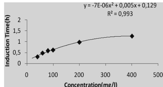
شکل ۵ رگرسیون چند جمله ای غلظت بر حسب زمان القاء در اسید تانیک
