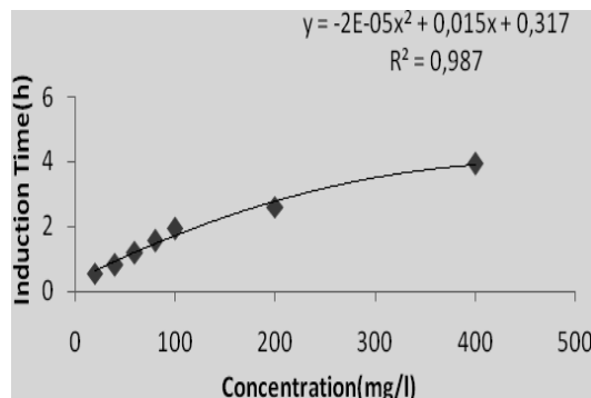
شکل ۱ رگرسیون چند جمله ای غلظت بر حسب زمان القاء در کوثرستین
