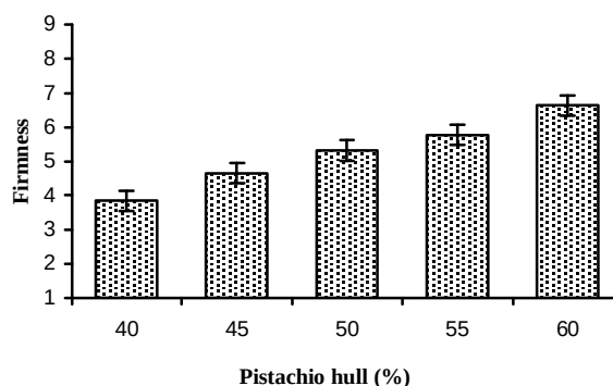
شکل 6 اثر درصد پکتین مورد استفاده بر سفتی مارمالاد پوست
