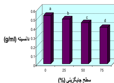
شکل 2 اثر سطوح جایگزینی wpc بر دانسیته
