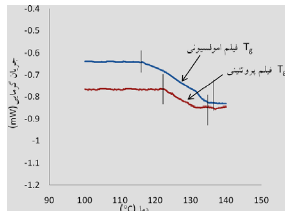
شکل ۴ دمای انتقال شیشه‌ای فیلم پروتئین گلوبولین پسته و فیلم امولسیونی حاوی ۶ درصد اسید استتاریک
