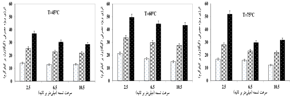
شکل ۲ مقادیر انرژی ویژه مصرفی برای خشک کردن میوه بنه در شرایط مختلف خشک‌کن پیوسته نیمه صنعتی (□ ۱ متر بر ثانیه، □ ۱/۵ متر بر ثانیه و ■ ۲ متر بر ثانیه)
