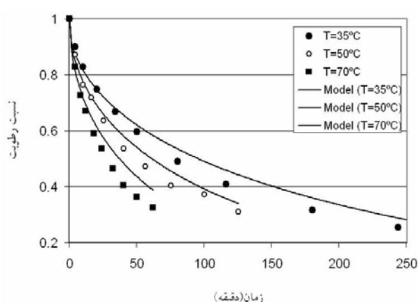
شکل ۱ مقایسه تغییر نسبت رطوبت در طی خشک شدن حاصل از داده های آزمایشگاهی و مدل کروی دانه گندم
