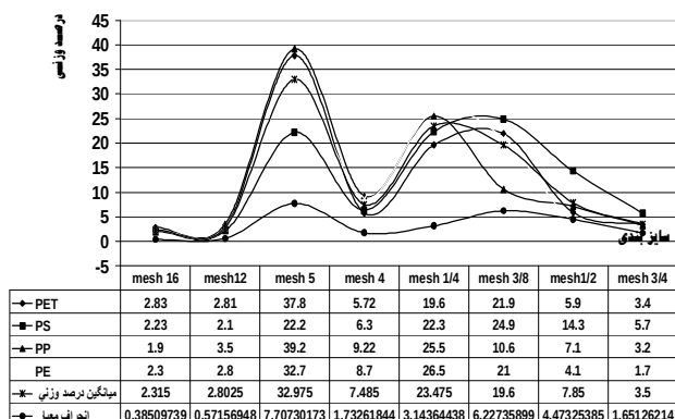
نمودار مقایسه ای درصد میانگین در صد وزنی مواد اولیه آسیابی
