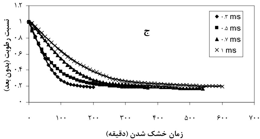
شکل ۱ تاثیر سرعت جریان هوا ( 0.3 \blacklozenge ، 0.5 \blacksquare ، 0.7 \blacktriangle و 1 \times متر بر ثانیه) بر نسبت رطوبت دانه‌های انار در فرآیند خشک شدن بر حسب میزان برازش داده‌ها با مدل میدیلی (خطوط پیوسته) در سه شدت تابش فروسرخ (الف) 22 \text{ W cm}^{-2} ، (ب) 31 \text{ W cm}^{-2} ، (ج) 49 \text{ W cm}^{-2}
