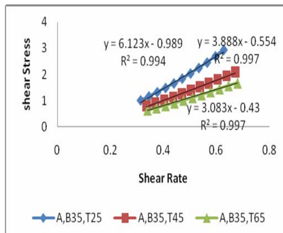
شکل ۴ رابطه سرعت برشی و تنش برشی شیر انگور در دمای °C ۲۵ و بریکس های مختلف
