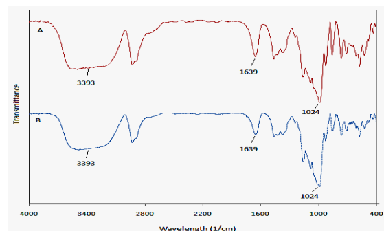
شکل ۲ طیف سنجی FT-IR نمونه های (A) نشاسته طبیعی گندم (B) نشاسته فسفریل گندم با درجه جایگزینی ۰/۰۹۶ درصد.
