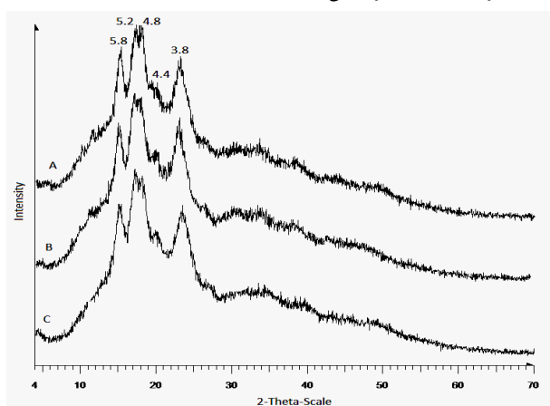
شکل ۴ الگوی XRD بدست آمده برای (A) نشاسته طبیعی، (B) نشاسته هیدروکسی پروپیل و (C) نشاسته فسفریل گندم.
