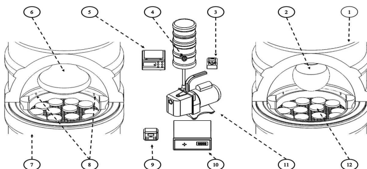
شکل ۱ نمای خشک کن آزمایشگاهی خلأ- مادون قرمز (۱-محفظه‌ی بالایی خشک کن، ۲- لامپ تنگستن، ۳- ترمومتر، ۴- سنسور فشار، ۵- ترازوی دیجیتال، ۶- لامپ کوارتز، ۷- محفظه‌ی پایینی خشک کن، ۸- سنسورهای k، ۹- ترموستات، ۱۰- سیستم کنترل فشار، ۱۱- پمپ خلأ و ۱۲- برش-های هلو)
