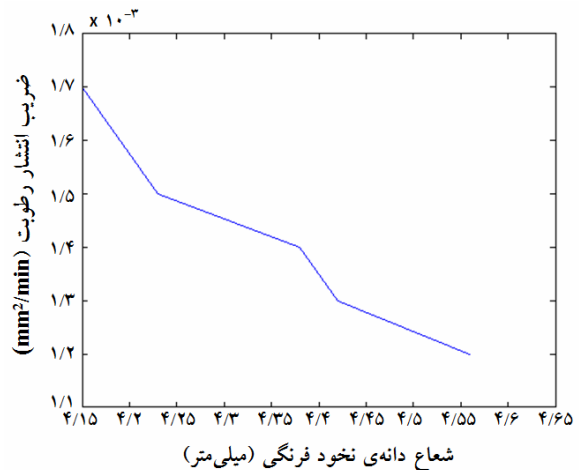
شکل ۲ نمودار ضریب انتشار رطوبت با شعاع دانه‌های نخود فرنگی در طول رطوبت‌افزایی در دمای ۵ درجه‌سانتی‌گراد
