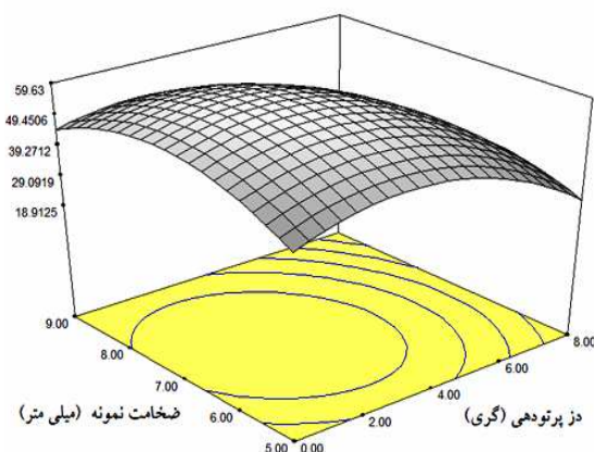
شکل ۶: تاثیر دز پرتودهی و ضخامت نمونه بر شاخص L^*
