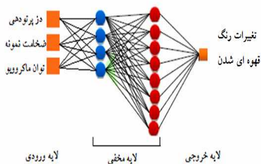
شکل ۱: دیاگرام بهترین مدل شبکه عصبی مصنوعی
