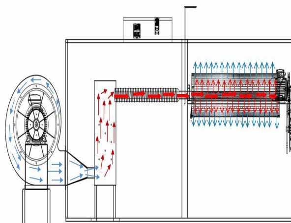
شکل ۲ نمای روبه‌رو و مسیر هوای داغ خشک‌کن
