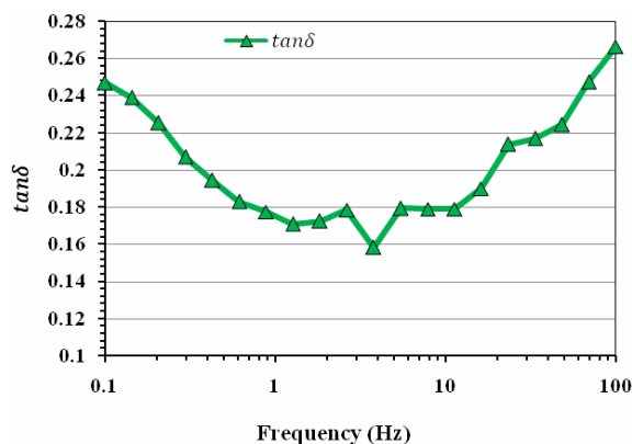
شکل ۴ تأثیر تغییرات فرکانس روی تانژانت افت (مثلت توپر) پنیر آروشه اندازه گیری شده در محدوده کرنش کمتر از ۲٪ در دمای ۲۵ درجه سانتیگراد
