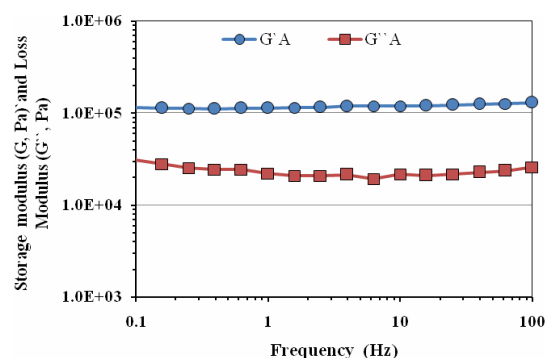
شکل ۳ تأثیر تغییرات فرکانس روی ضرایب الاستیک (دایره توپر)، افت (مربع توپر) پنیر آروشه اندازه گیری شده در محدوده کرنش کمتر از ۲٪ در دمای ۲۵ درجه سانتیگراد
