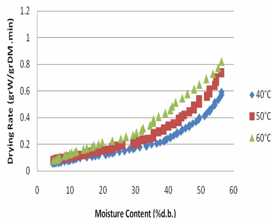
شکل ۱۰ نرخ خشک شدن در سرعت چرخش ۵rpm
