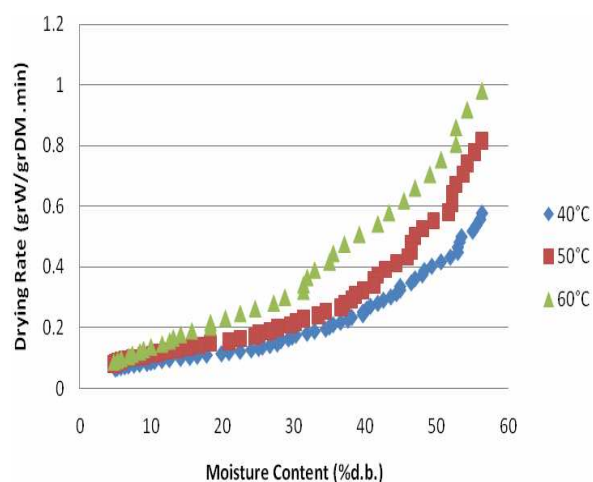
شکل ۱۲ نرخ خشک شدن در سرعت چرخش ۱۵rpm
