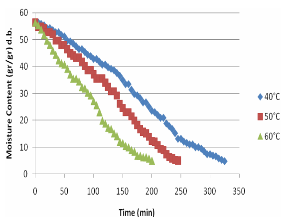
شکل ۷ منحنی رطوبت-زمان در دماهای متفاوت، سرعت چرخش ۵ rpm
