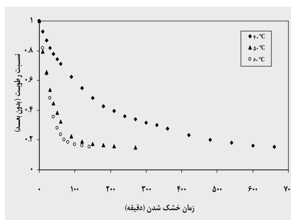
شکل ۸ تغییرات نسبت رطوبت بر حسب زمان در سطوح مختلف
