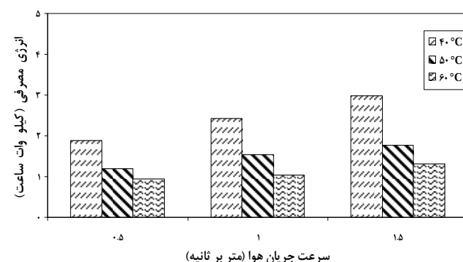
شکل ۹ انرژی مصرفی خشک کردن آلوده و با چرخه ۵۰٪ بازگردش هوای گرم
