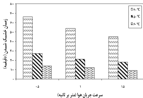
شکل ۲ زمان خشک شدن آلوده ورا تحت شرایط مختلف خشک شدن در حالت ۵۰٪ بازگردش جریان هوای گرم
