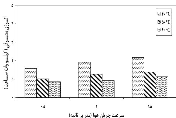
شکل ۱۰ انرژی مصرفی خشک کردن آلوده و با چرخه ۷۵٪ بازگردش هوای گرم
