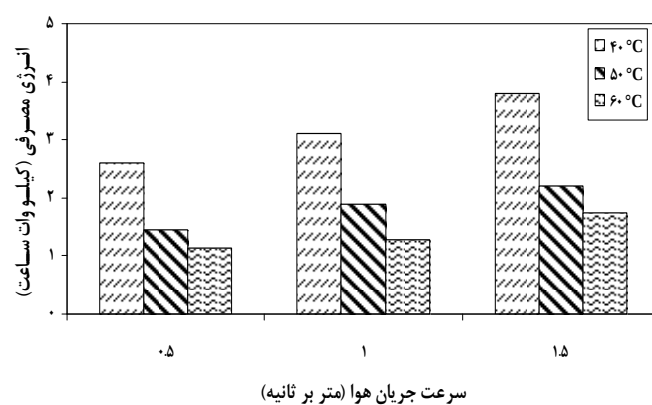
شکل ۸ انرژی مصرفی خشک کردن آلوده و با چرخه بدون بازگردش هوای گرم
