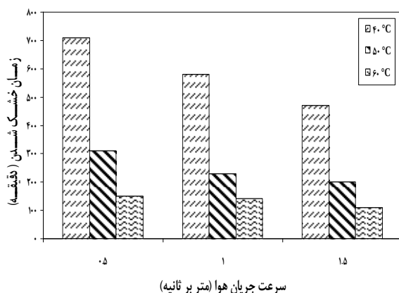
شکل ۳ زمان خشک شدن آلوده ورا تحت شرایط مختلف خشک شدن در حالت ۷۵٪ بازگردش جریان هوای گرم
