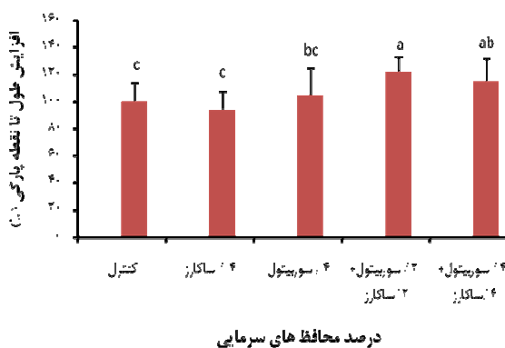
شکل ۳ افزایش طول تا نقطه پارگی فیلم های حاصل از پروتئین ماهی در حضور محافظ های سرمایی
