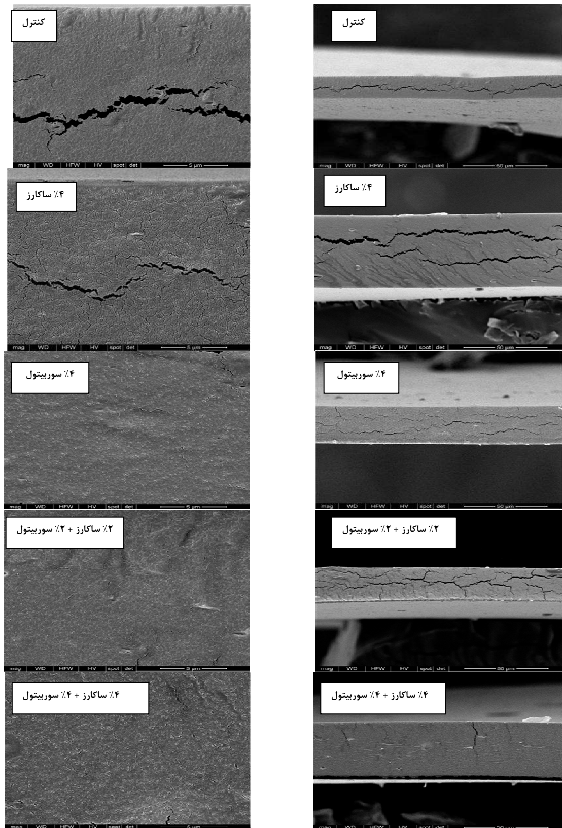
شکل ۵ ساختار میکروسکوپ الکترونی فیلم های تهیه شده از پروتئین ماهی در حضور محافظ های سرمایی. تصاویر سمت چپ مربوط به سطح فیلمها (بزرگنمایی \times 10000 ) و تصاویر سمت راست مربوط به برش عرضی فیلم ها (بزرگنمایی \times 1000 ) است.
