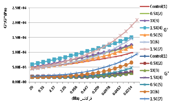
نمودار ۱۲ آزمون طیف فرکانسی بر روی خمیرهای فاقد گلوتن و تأثیر هیدروکلوئیدها بر G' و G'' به صورت جداگانه (۲۰-۰/۰۱-۳۰ Hz)
