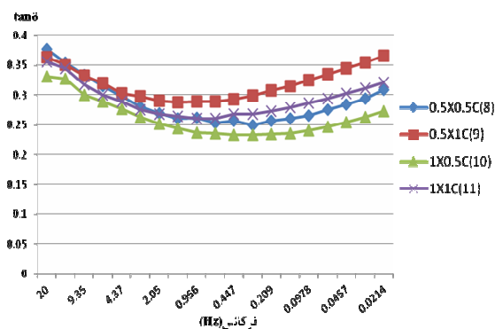
نمودار ۱۶ آزمون طیف فرکانسی بر روی خمیرهای فاقد گلوتن و تأثیر تلفیقی هیدروکلوئیدها بر \tan\delta (۲۰ Hz - ۳۰۰,۰/۰۱)
