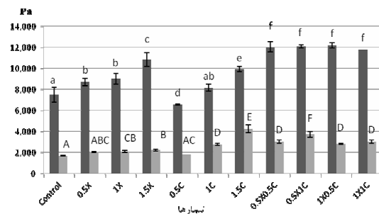
نمودار ۱۴ مقایسه تأثیر تیمارهای تلفیقی صمغ‌ها و تیمارهای حاوی صمغ به تنهایی بر G' و G'' در فرکانس ۱ Hz ( P \geq 0.05 )
