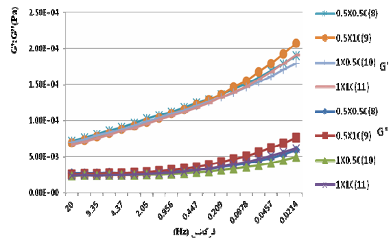
نمودار ۱۳ آزمون طیف فرکانسی بر روی خمیرهای فاقد گلوتن و تأثیر تلفیقی هیدروکلوئیدها بر G' و G'' (۲۰ Hz - ۳۰۰,۰/۰۱)
