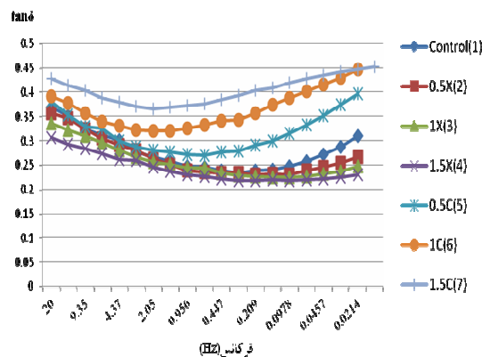
نمودار ۱۵ آزمون طیف فرکانسی بر روی خمیرهای فاقد گلوتن و تأثیر هیدروکلوئیدها بر \tan\delta به صورت جداگانه (۲۰ Hz - ۳۰۰,۰/۰۱)
