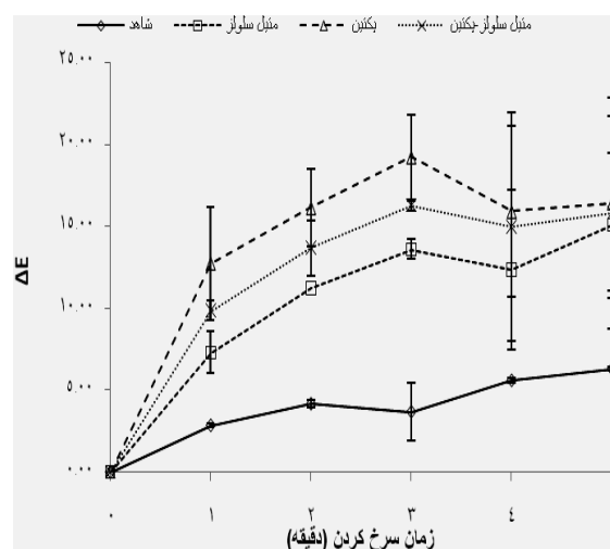
نمودار ۳ میانگین مقدار ΔE در طول دوره سرخ کردن فلافل
