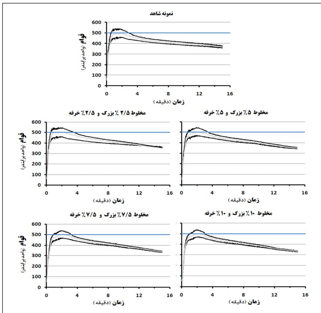
شکل ۲ منحنی‌های فارینوگرام آرد شاهد و آردهای غنی شده با درصدهای مختلف مخلوط بزرگ و خرفه. شکل‌های ارائه شده منحنی‌های میانگین سه بار اندازه‌گیری می‌باشند.
