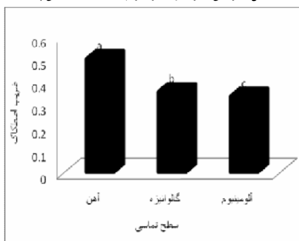
شکل ۳ بررسی تأثیر تماسی بر ضریب اصطکاک استاتیکی پسته
