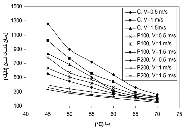
شکل ۱ تاثیر دما و سرعت هوا بر زمان لازم برای خشک کردن دانه های انار
