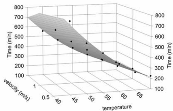
شکل ۶ تاثیرات دما و سرعت هوا بر زمان خشک شدن دانه انار با استفاده از پیش تیمار مایکروویو ۱۰۰ وات
