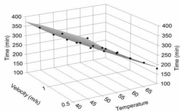
شکل ۷ تاثیرات دما و سرعت هوا بر زمان خشک شدن دانه انار با استفاده از پیش تیمار مایکروویو ۲۰۰ وات
