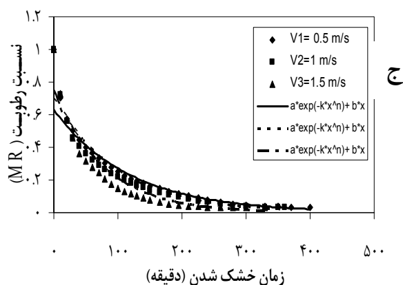
شکل ۴ منحنی های خشک شدن لایه نازک دانه انار در دمای ۴۵ درجه سلسیوس در الف) تیمار شاهد ب) تیمار مایکروویو با توان ۱۰۰ وات ج) تیمار مایکروویو با توان ۲۰۰ وات و به همراه خطوط پیشگویی شده توسط مدل تبدیلی در سرعت‌های مختلف هوا
