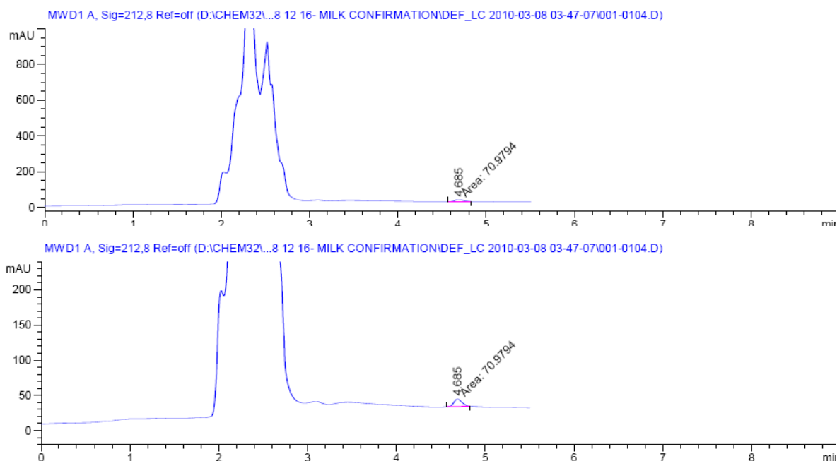
شکل ۲ کروماتوگرام نمونه شیر پاستوریزه مشکوک به وجود کلوتریمازول، جهت وضوح بیشتر، کروماتوگرام دوم بزرگمایی شده کروماتوگرام اول است.
