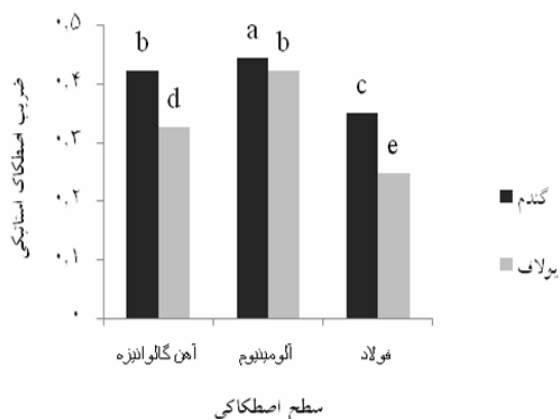
شکل ۱۴ میانگین اثر متقابل نوع دانه و سطح اصطکاکی برای ضریب اصطکاک استاتیکی
