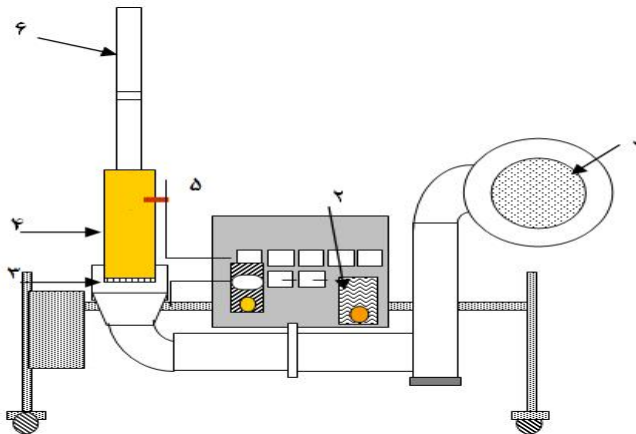
شکل ۲ طرح‌واره تونل باد مورد استفاده در تحقیق
