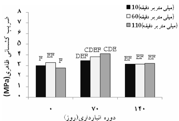
شکل ۳ میانگین اثر متقابل سه تایی جهت بارگذاری، دوره انبارداری و سرعت بارگذاری بر ضریب کشسانی ظاهری سیرچه کامل به ترتیب هنگام بارگذاری در راستای عرضی (بالا) و در راستای ضخامت (پایین) در دوره انبارداری ۰، ۷۰ و ۱۴۰ روز پس از برداشت
