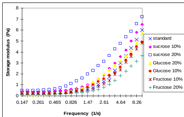
شکل ۸ تأثیر شیرین‌کننده‌های طبیعی بر روی مدول G' ذخیره محلولهای گوار ۰/۵٪
