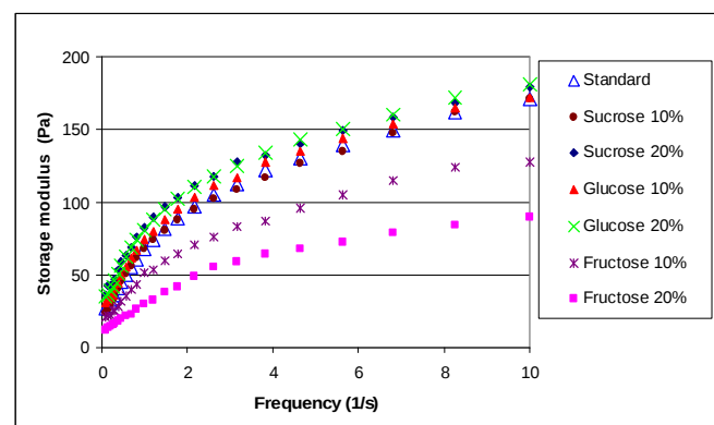
شکل ۷ تأثیر شیرین‌کننده‌های طبیعی بر روی مدول ذخیره G' محلولهای گوار ۱/۵٪
