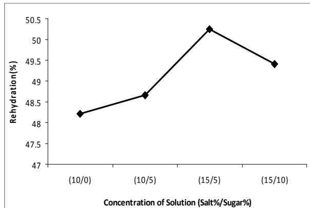
نمودار ۲ اثر غلظت محلول اسمزی بر درصد بازجذب آب.
