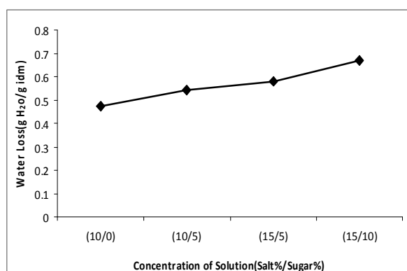
نمودار ۵ اثر غلظت محلول اسمزی بر میزان اتلاف آب.
