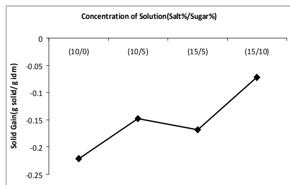
نمودار ۶ اثر غلظت محلول اسمزی بر میزان جذب مواد جامد.
