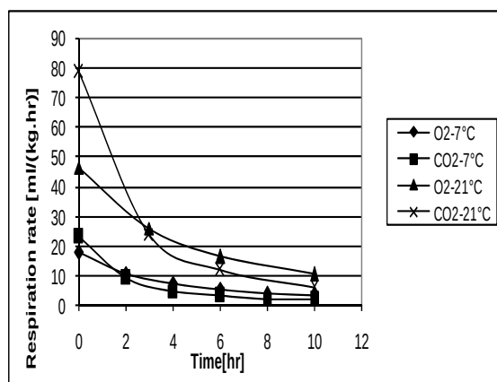
شکل ۵ سرعت تنفس هویج هلی کل در دمای آزمایشگاه و یخچال
