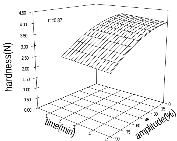
نمودار 1 تاثیر شدت و مدت زمان اعمال صوت بر سفتی بافت نان حاصل از گندم سن زده 2 ساعت بعد از پخت
