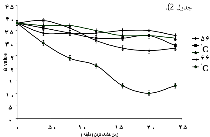
شکل 6 تاثیر دما و زمان بر پارامتر (a) رنگ رطب در طی خشک کردن
