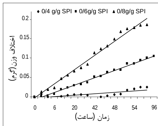
شکل 3 تغییرات وزنی ایجاد شده در فیلم‌های ایزوله پروتئینی سویا بر اثر جذب بخار آب در طی 96 ساعت نگهداری
