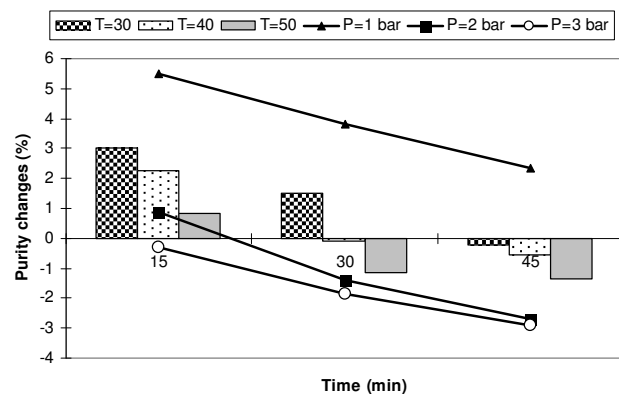
شکل ۲ تغییرات دینامیکی درجه خلوص تراوه در دماها و فشارهای مختلف فرآیند اولترافیلتراسیون شربت رقیق چغندر
