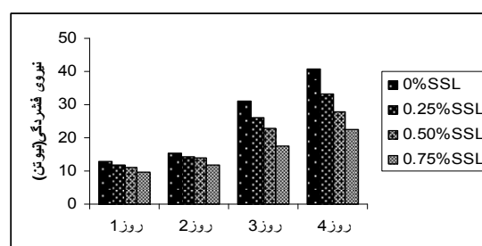
نمودار ۳ آزمون فشردگی نان های تافتون در روزهای ۱، ۲، ۳ و ۴
