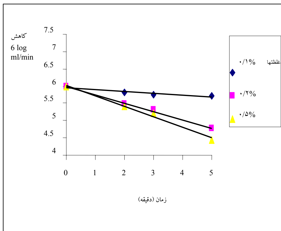
شکل ۱ منحنی بقا برای مخمر ساکرومسیس سرویزیه با استفاده از اسانس لیمونین در غلظت‌های ۱/۲ و ۵/۰ درصد
