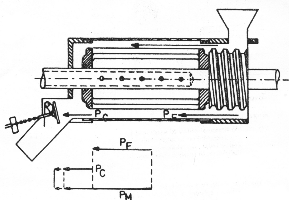
شکل ۱ نمایی از سفیدکن مالشی دمشی - مقدار فشار دهانه تخلیه دستگاه
