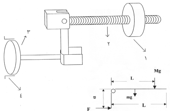
شکل ۳ مکانیزم وزنه و لنگ: ۱- وزنه ۲- پیچ هادی ۳- دریچه ۴- دهانه تخلیه دستگاه سفیدکن
