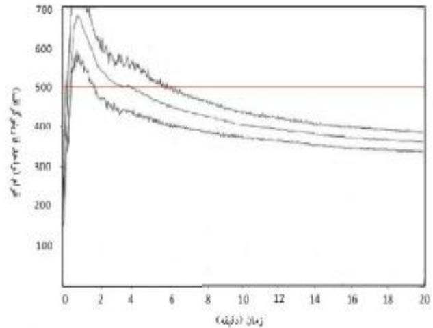
شکل 5 منحنی فارینوگرام خمیر هیدراته در دمای 25 °C به مدت 1/5 ساعت
