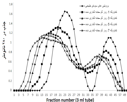
شکل ۲ کروماتوگرام پروتئین های سویا و کنژوگه ها
