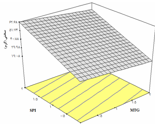
شکل ۶ تغییرات سختی نمونه‌های بستنی در اثر تغییرات مقدار SPI و MTG
