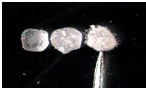
شکل ۵ مقایسه بلور اسید سیتریک تیمار نشده (چپ)؛ اسید سیتریک آغشته به کربوکسی متیل سلولز رشته ای (وسط)؛ بلور اسید سیتریک پوشش دار شده با کربوکسی متیل سلولز رشته ای (راست) توسط امواج مایکروویو در مدت ۳۰۰ ثانیه (تصویربرداری شده توسط دوچشمی آزمایشگاهی با بزرگ نمایی ۱/۵).
