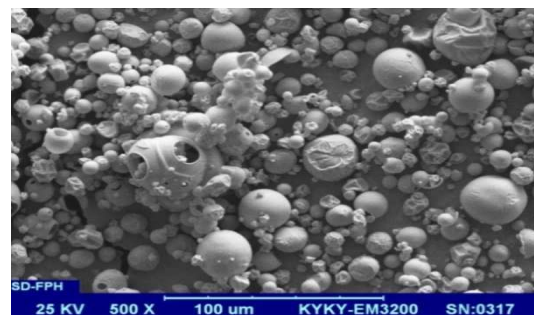
شکل ۴ تصویر میکروسکوپ الکترونی از پودر پروتئین هیدرولیز شده گوشت کوسه چانه سفید (۵۰۰×)
