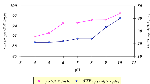
نمودار ۱ تأثیر pH بر زمان فیلتراسیون و درصد رطوبت کیک لجن
