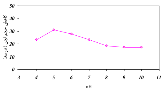
نمودار ۳ تأثیر pH بر درصد کاهش حجم لجن
