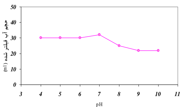
نمودار ۲ تأثیر pH بر حجم آب فیلتر شده در زمان ثابت
