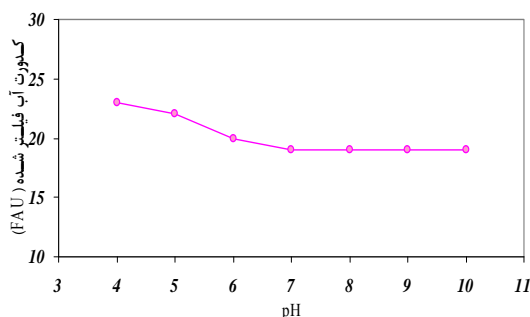
نمودار ۴ تأثیر pH بر کدورت آب فیلتر شده
