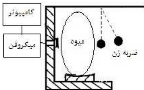
شکل ۱ سامانه صوتی
