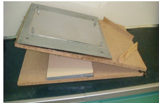
شکل ۱ دستگاه اندازه‌گیری ضریب اصطکاک استاتیکی
