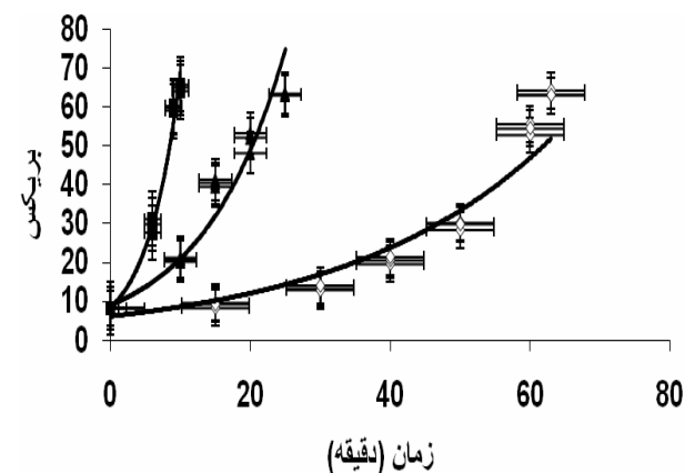
شکل ۱ تغییرات غلظت ایجاد شده با روش‌های مختلف تغلیظ (◇) حرارت تحت فشار اتمسفر، ▲ حرارت در اوپراتور چرخان تحت خلا، ■ حرارت در میکروویو و □ مدل پیش بینی شده)
